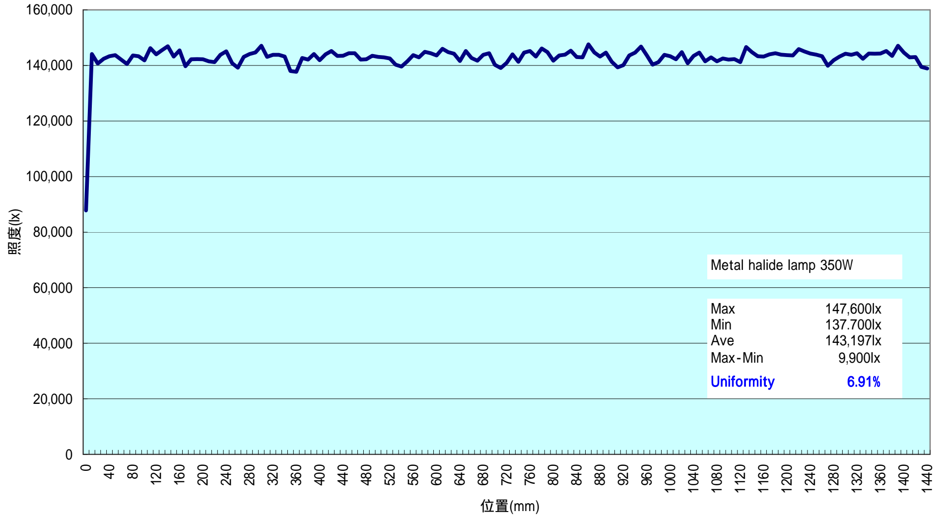
ラインライトガイド照度測定(w1448)
